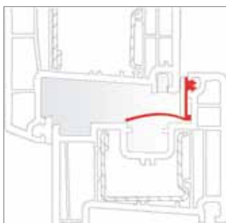
Blīvējuma pozīcija pie normāla gaisa spiediena
